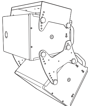
MCP50-X40 クラスタプレート上に MTB-X40ブラケットを使用した 50° の垂直クラスタ
