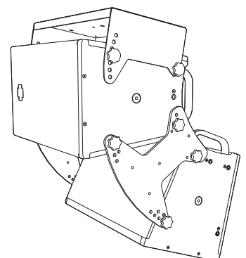
MCP70-X40 クラスタプレート上に MTB-X40 ブラケットを使用した 70° の垂直クラスタ
