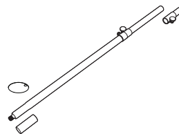
MPK-POLE 35MM M20ポールキット PAS-M20アダプタスリーブ付属 (単体別売可)
