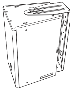
MUB-X40 Uプレート垂直方向壁取付例
