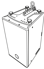
MTC-X40トップチャンネルおよび MPC50-X40クラスタプレート
