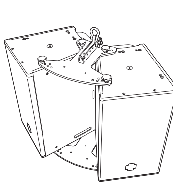
MCP70-X40 クラスタプレート上に MTC-X40トップチャンネルを使用した 70° 水平クラスタ
