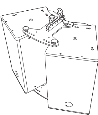
MCP50-X40 クラスタプレート上に MTC-X40トップチャンネルを使用した 50° の水平クラスタ
